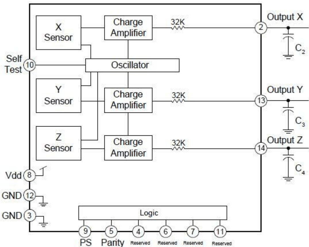
&lt;KXM52のブロックダイアグラム&gt;
