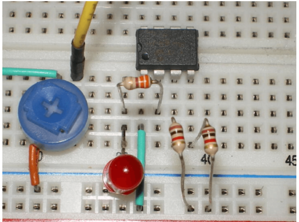
湿度スイッチがOFFの状態
